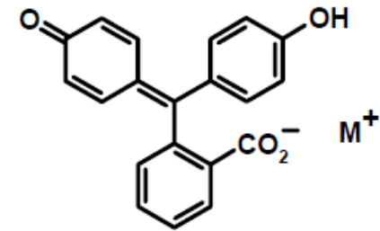
Phenolphthalein (nicht fluoreszent)
